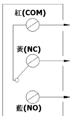
流量減少時開關動作情況
