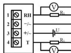
三線式電壓型溫濕度傳訊器
