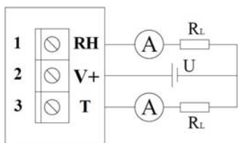
二線式溫濕度傳訊器
