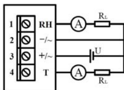
三線式電流型溫濕度傳訊器
