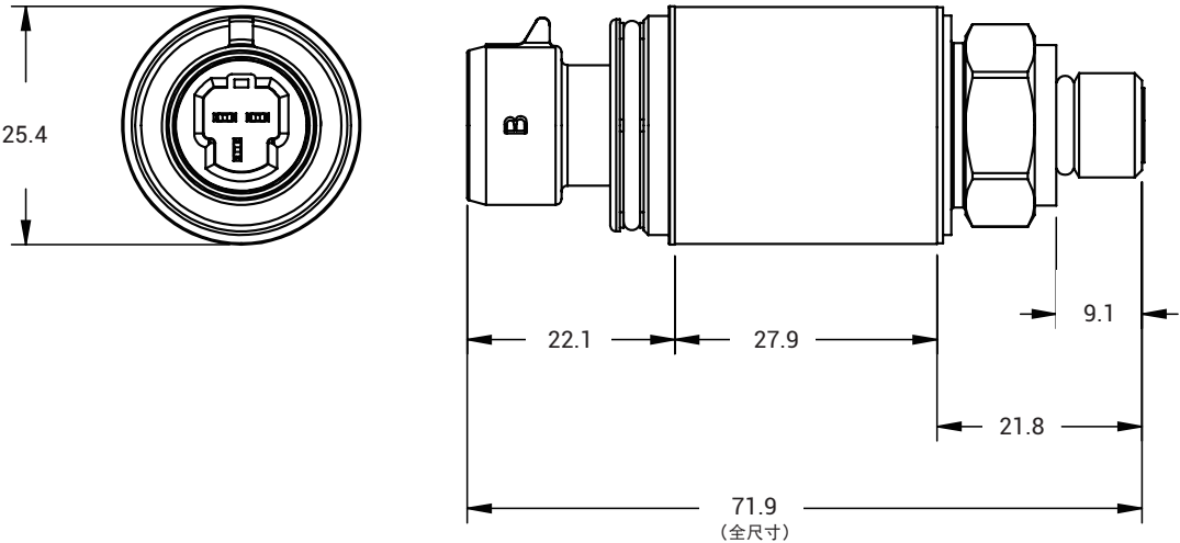
*图示为7/16" SAE外螺纹接口 (J7) 和3针Packard接口 (P1)。
