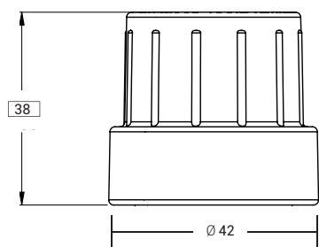
安装导管盖
