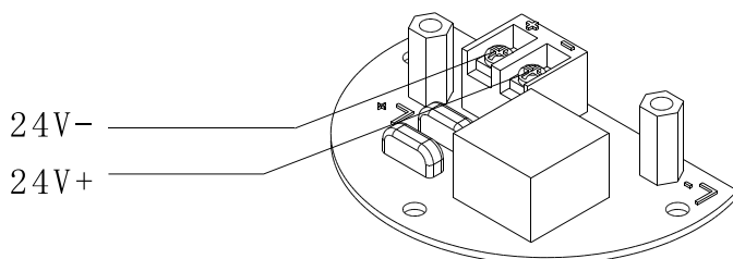
DC 4~20mA(二線)
