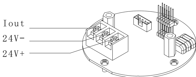
DC 4~20mA(三線)
