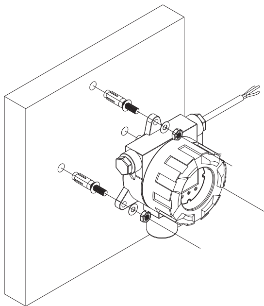
壁掛式安裝
