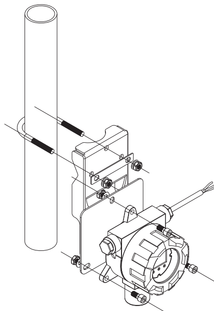
管道式安裝
